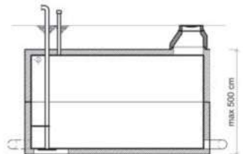
Variante 2: zweischalig
