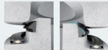
Gleitringsdichtung SG Lastübertragungsring TSB
