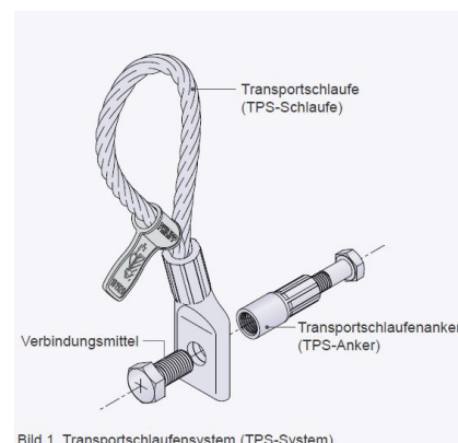
Bild 1 Transportschlaufensystem (TPS-System)
