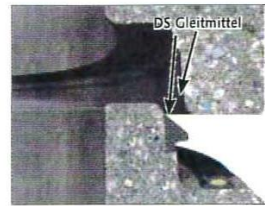
Beispiel: lose Schachtdichtung
