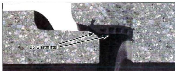
Beispiel: integrierte Rohrdichtung
