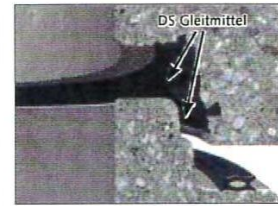
Beispiel: integrierte Schachtdichtung
