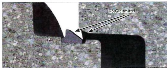
Beispiel: Gleitringdichtung in einer Kammer auf dem Spitzende
